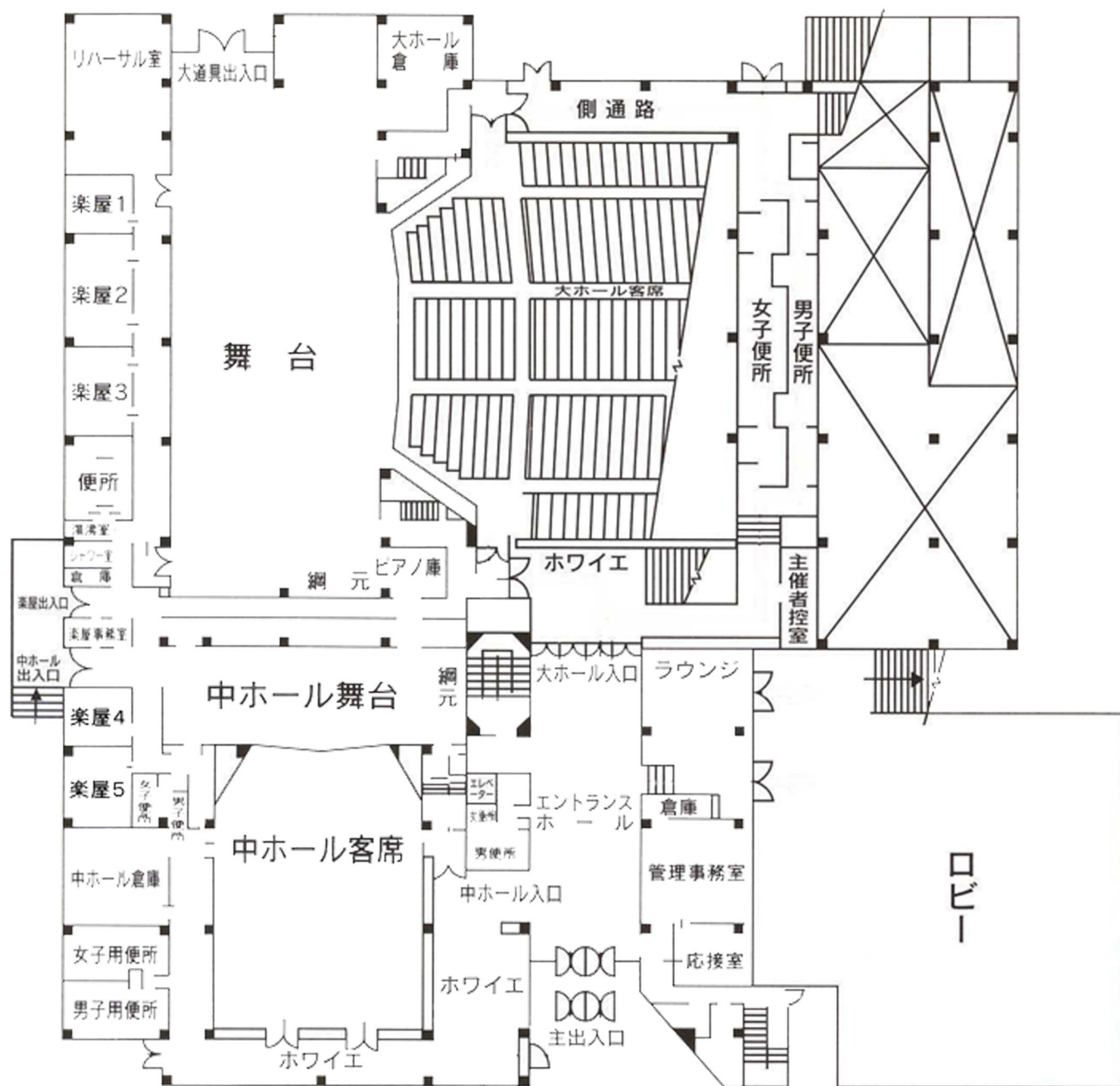
一階平面図
