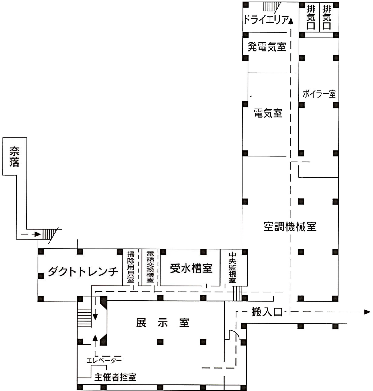
地階平面図 (点線は避難経路)
